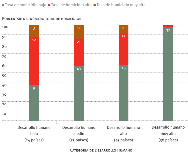
FIGURA 5.2 Desagregación de datos sobre la violencia homicida en 182 países según el IDH, 1986–2009
